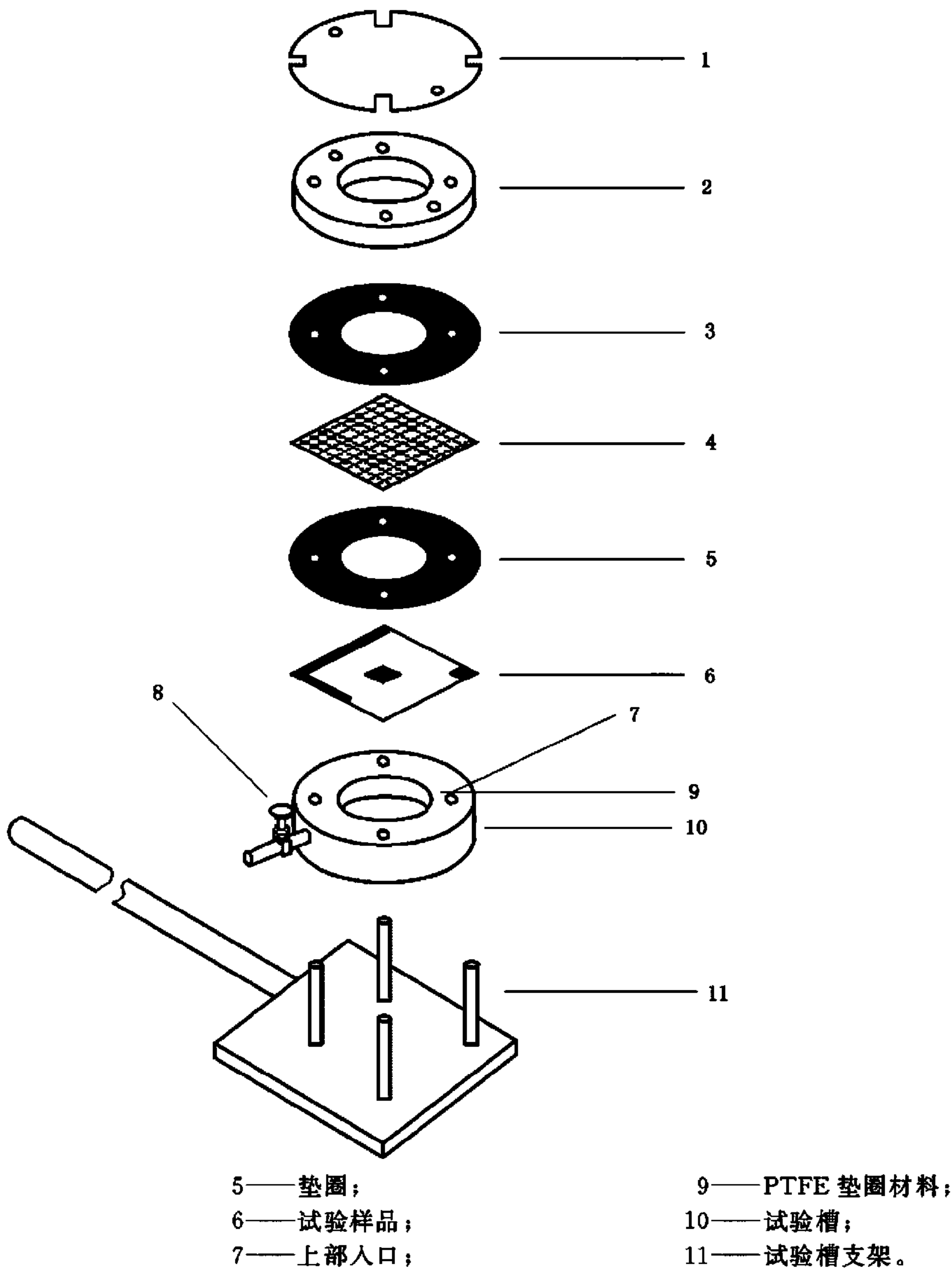
图 A.1 试验槽结构
